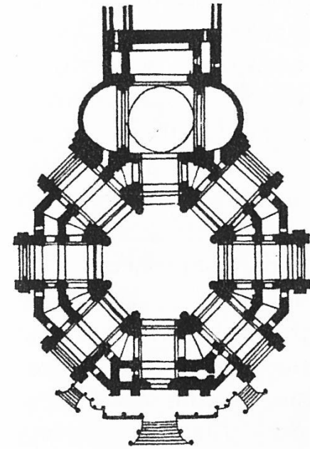
KOŚCIÓŁ FILIPINÓW W GOSTYNIU.
