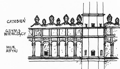
ATTYKA NA RATUSZU POZNAŃSKIM Z 1561 R.
