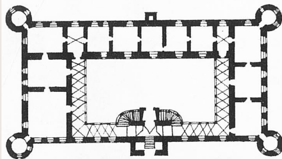
PLAN ZAMKU W BARANOWIE
