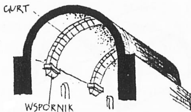
SKLEPIENIE KOLEBKOWE NA GURTACH
