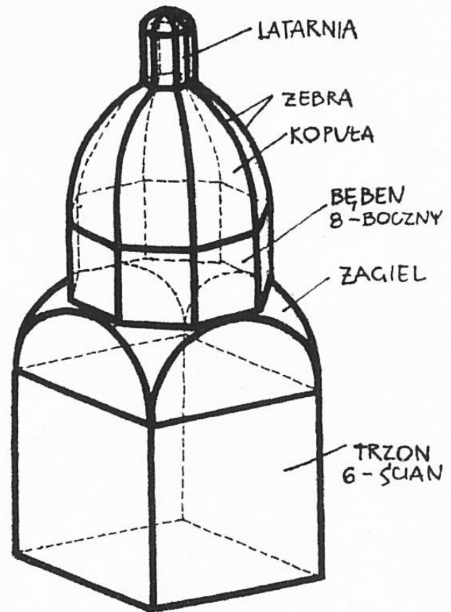
SCHEMATYCZNA BRYŁA KAPLICY ZYG MUNTOWSKIEJ
